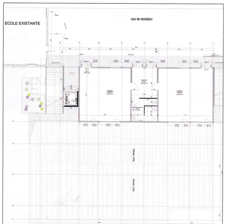
Plan intérieur de l'agrandissement du haut de l'école
